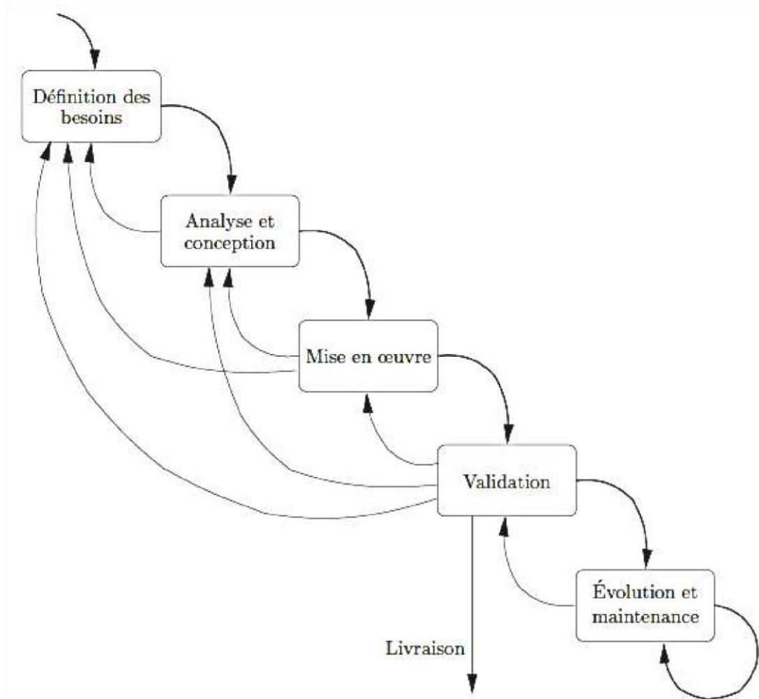
Modèle du cycle de vie en cascade Incontrôlable
