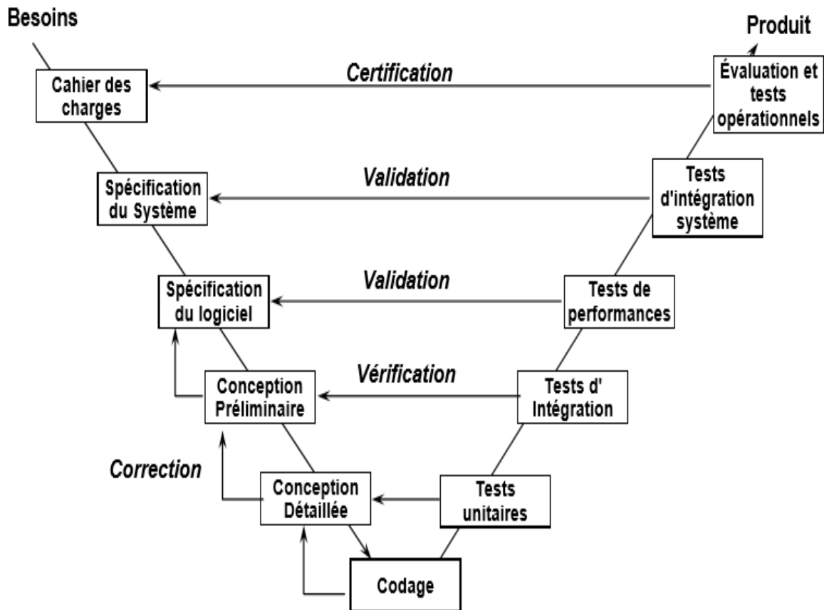
Modèle du cycle de vie en « V » N° 2
